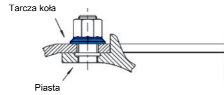
Centrowanie na piaście
