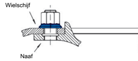
Naaf centrering
